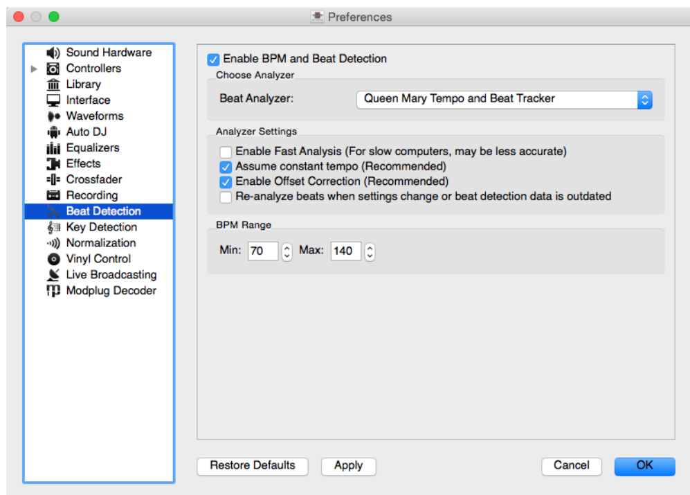
Figure2: Prefències del Mixxx - Opcions de BPM
