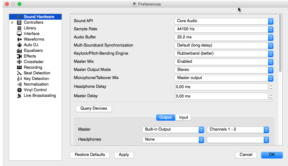
Figure2: Preferències de maquinari de so del Mixxx
