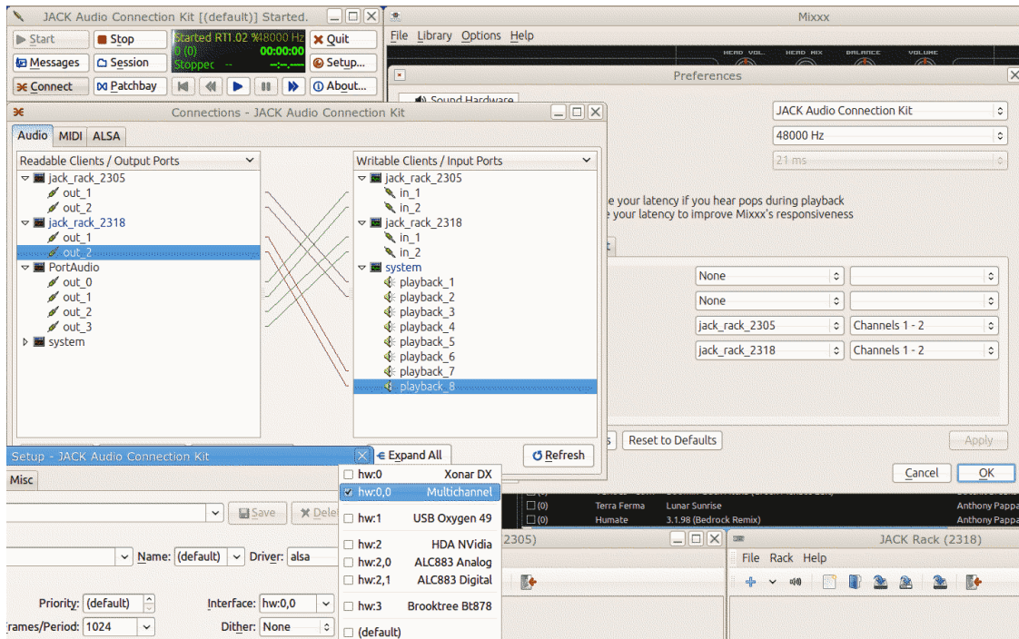
Figure3: Enrutament amb el JACK per a efectes externs a GNU/Linux
